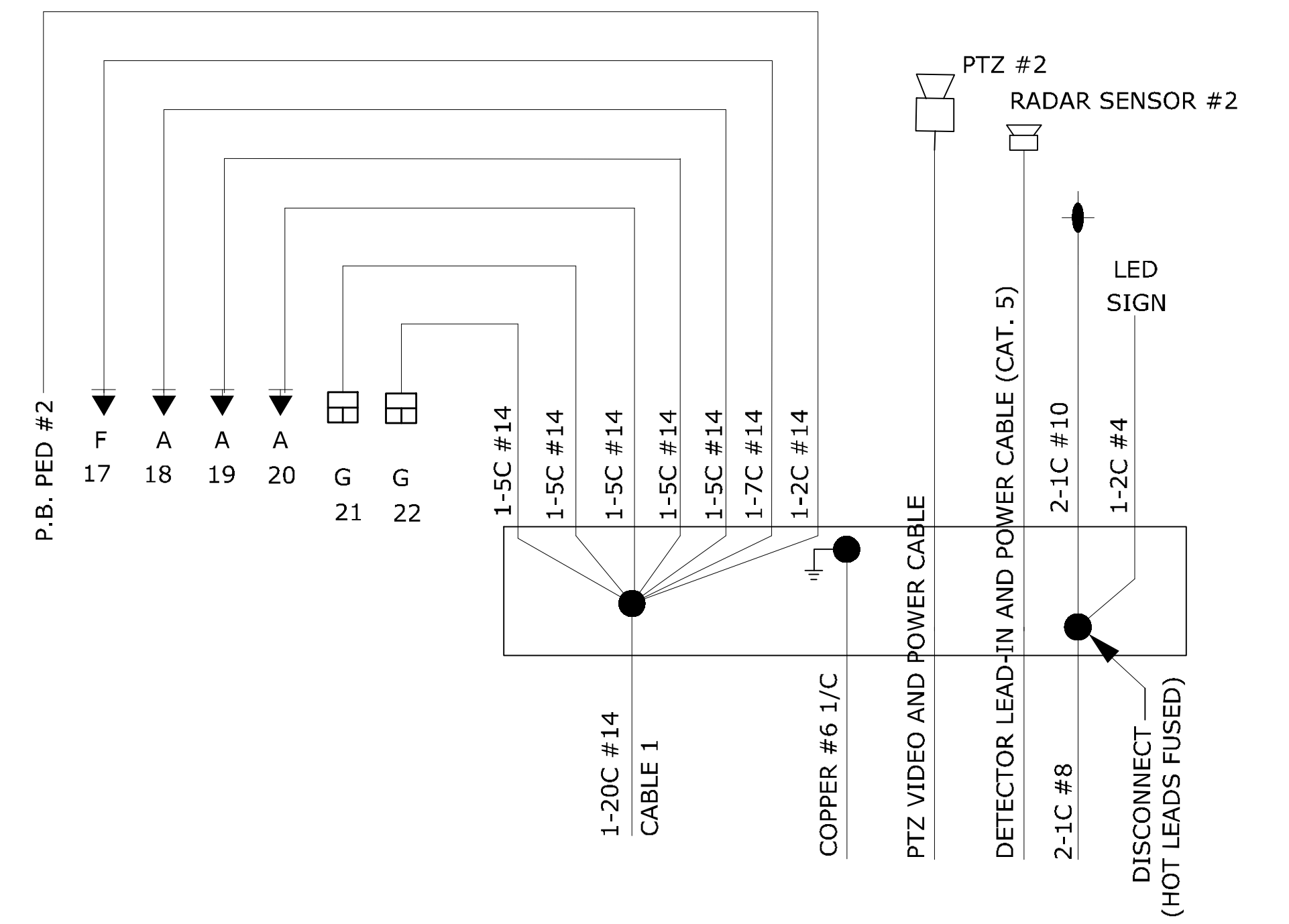
POLE #2
